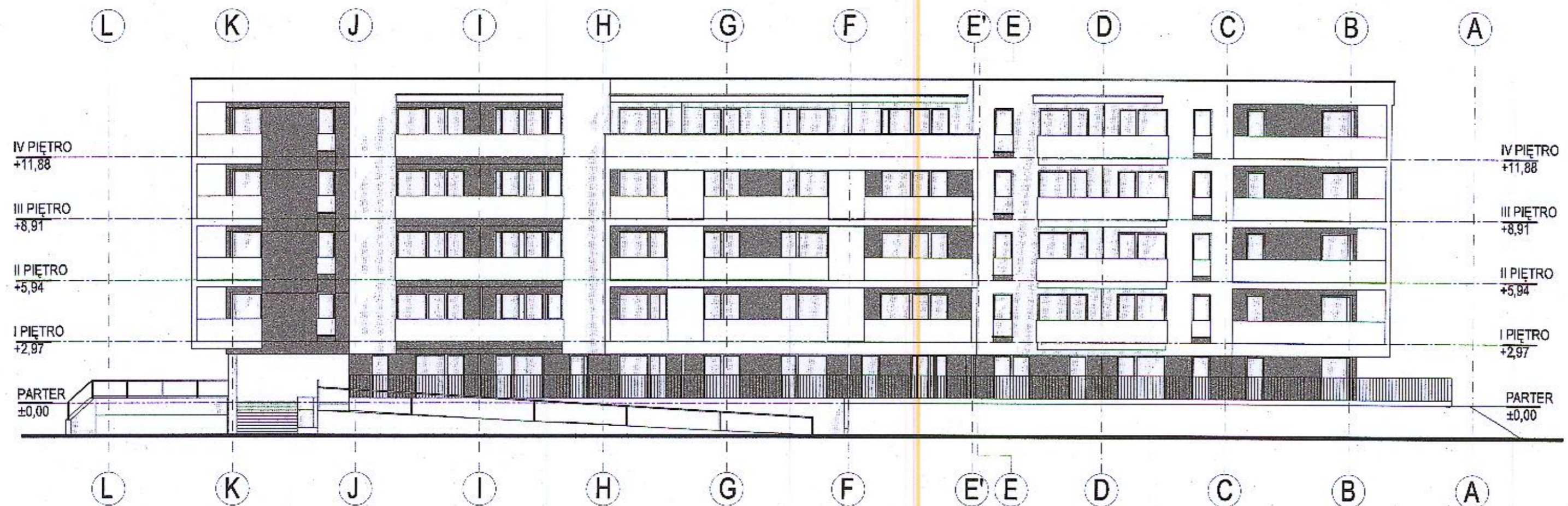
ELEWACJA POŁUDNIOWO-WSCHODNIA
